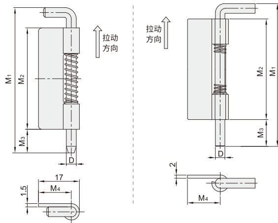
单页弹簧型 VKY25/26
