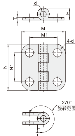
台阶型 VKH46
