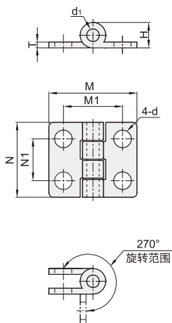
长板型 VKH45
