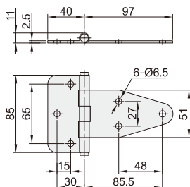
长板型 VKH45
