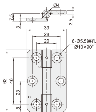
台阶型 VKH46
