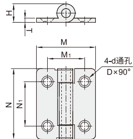
VKH21 规格: 5032
