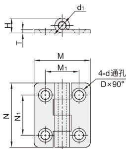
VKH11 4孔安装
