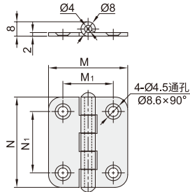
VKH16 4孔安装
