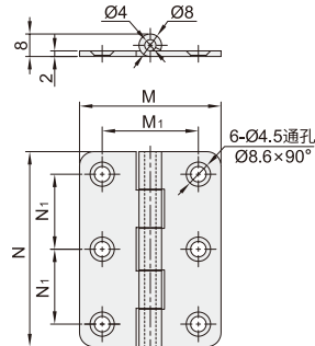
VKH16 6孔安装
