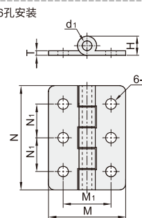
6孔安装
