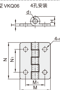
圆孔型 VKQ06
