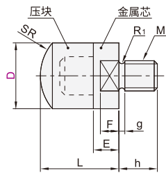
圆型 MWAL31/32
