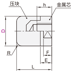
平型 MWAL01/02
