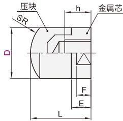
圆型 MWAL11/12
