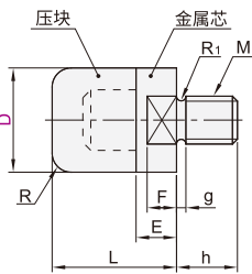
平型 MWAL21/22
