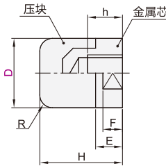
平型 MWAN51/52/53/54/55
