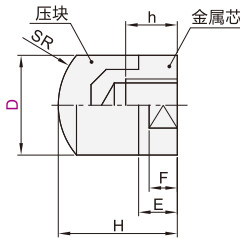
圆型 MWAN61/62/63/64/65
