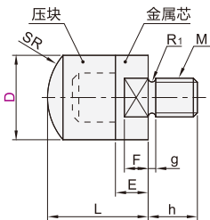
圆型 MWAN81/82/83/84/85
