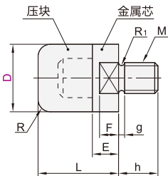
平型 MWAN71/72/73/74/75
