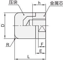
平型 MWAN01/02
