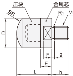
圆型 MWAN31/32
