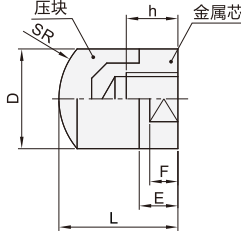
圆型 MWAN11/12
