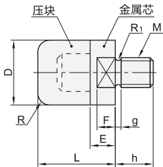
平型 MWAN21/22
