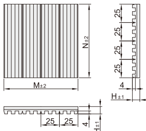
突起详图
