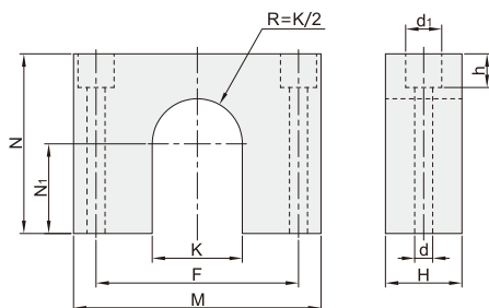
标准型 MWAF05
