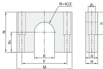
薄壁型 MWAF06
