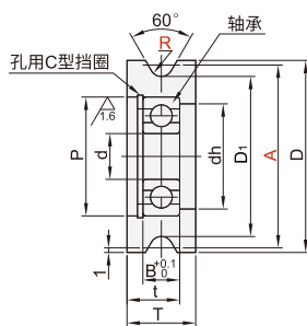
标准型 VB Y01/02/11/21
