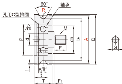
外螺纹型 VB Y51/52/61/71
