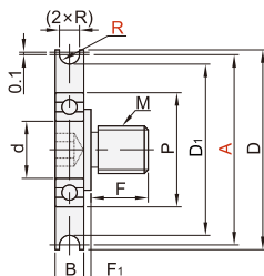
外螺纹型 VB51/52/61/71
