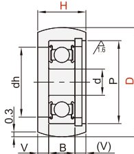
圆弧型 VBG21/22/24/31/36
