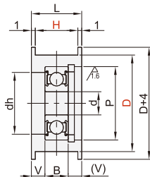
法兰型 VBG01/02/04/11
