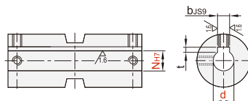
■键槽孔+螺孔型
