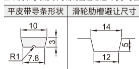
■平皮带导条形状与滑轮肋槽避让尺寸参考图
