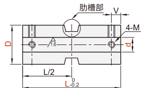
■圆孔+螺孔型
