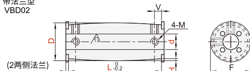
带法兰型 VBD02
