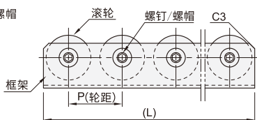
U型螺帽
