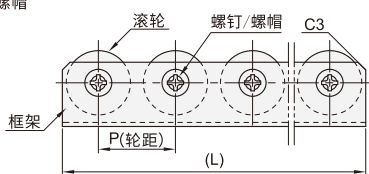
标准螺帽
