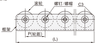
标准螺帽
