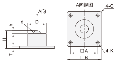
方法兰式 LFA20/22/24/26/28
