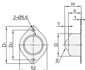
菱形法兰式-中载型 LFA06
