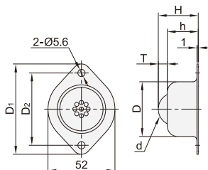
菱形法兰式-中载型 LFA07
