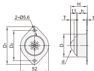
菱形法兰式-重载型 LFA08
