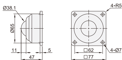
方法兰式-重载型 LFA09
