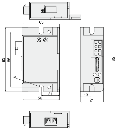
驱动器 BLD11
