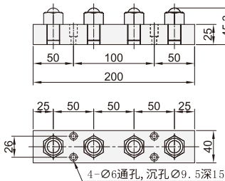
六角螺栓型 LFK05
