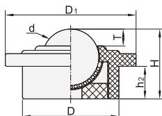
压入式 LFJ01
