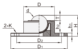
嵌入型 LFH31
