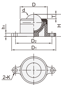
窄耳型 LFH11-25
