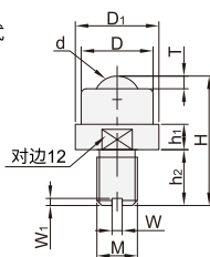
螺杆式 LFJ11
