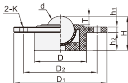
标准型 LFH01
