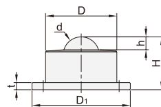
带弹簧向上使用型 LFE34
