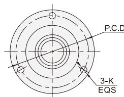
快速安装型:LFE73/74
