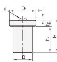
快速安装型:LFE73/74
