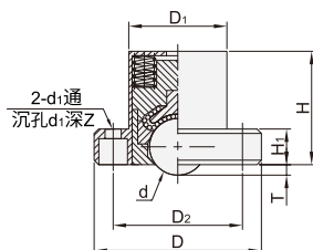
带弹簧向下使用型 LFE72
