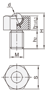
六角螺栓型 LFE01(S45C)
