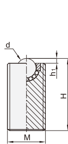
全螺纹型 LFE16(S45C)
