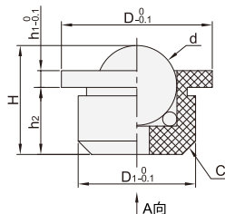
粘接式 LFC23
