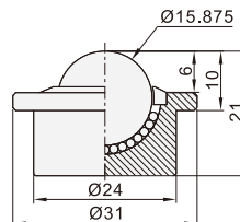
重型 LFB06/07-15
