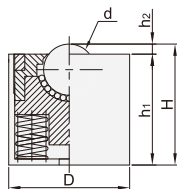
圆柱式·带弹簧 LFE71
