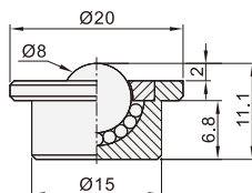
重型 LFB06/07-8
