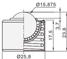
标准型 LFB01-15
