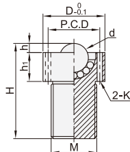
螺栓固定型 LSZ02
