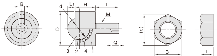
螺帽固定型 LSZ01(附带螺帽)
