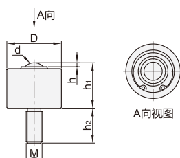
挡圈固定向下使用型 LSZ03
