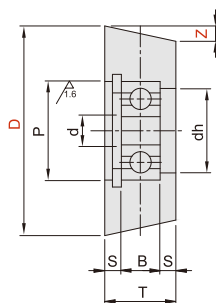
锥型
