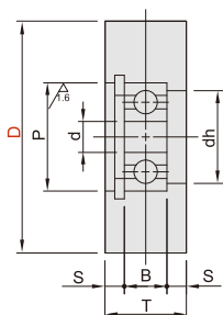
平头型
