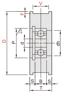
双法兰型
