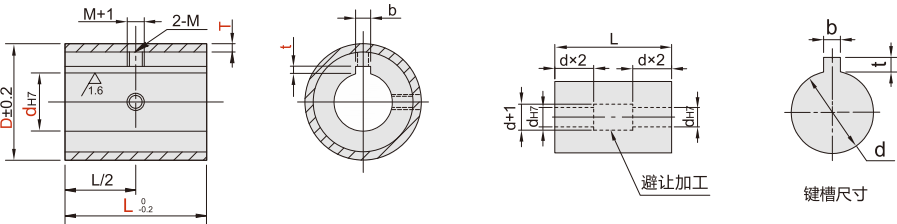
带螺纹孔式
