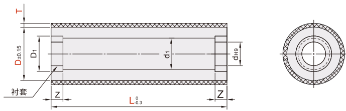
直柱形 LBH01 LBH02
