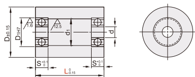
带轴承型 直柱形 LBG01/LBG02/LBG03/LBG04
