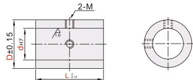
带止动螺丝型 直柱形 LBF03/LBF04
