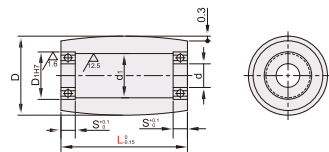
带轴承型 圆弧形 LBG31/LBG32/LBG33/LBG34
