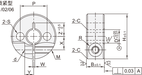
双螺孔锁紧型 SBJ51/52/56
