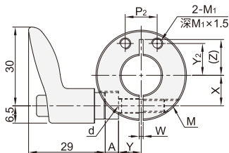
小型把手 SBT31/32/36
