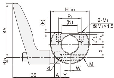
切割型 标准把手 SBT01/02/06
