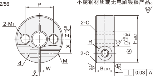
双螺孔锁紧型 SBJ51/52/56
