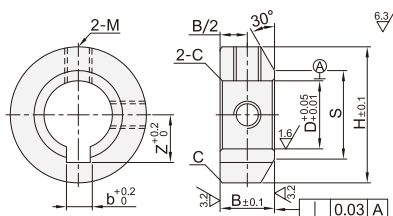
避空键槽型 SBR01/02
