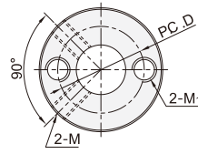
双螺孔型 SBC51/52/56
