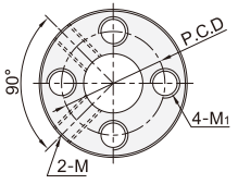
四螺孔型 SBC81/82/86
