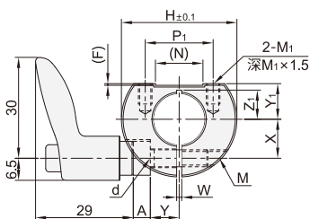
小型把手 SBT11/12/16
