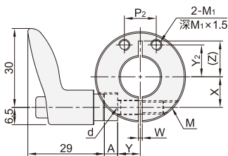
小型把手 SBT31/32/36
