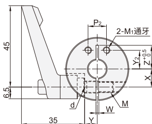
侧安装型 标准把手 SBY41/42/46
