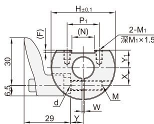
小型把手 SBY31/32/36
