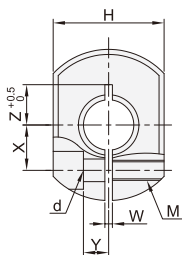
分离型.紧定螺钉锁紧型 SBS61/62/66
