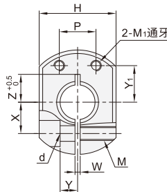
开口型.侧安装型 SBS21/22/26
