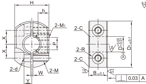
分离型.紧定螺钉锁紧型 SBS61/62/66
