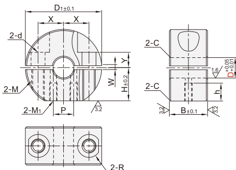
分离型 SBW41/42/46/51
