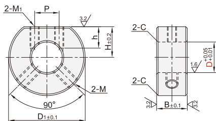
分离型 SBW41/42/46/51
