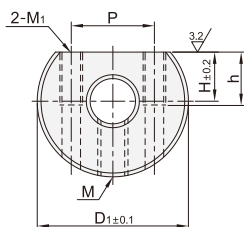
开口型 SBW21/22/26/31
