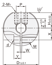
开口型 SBW21/22/26/31
