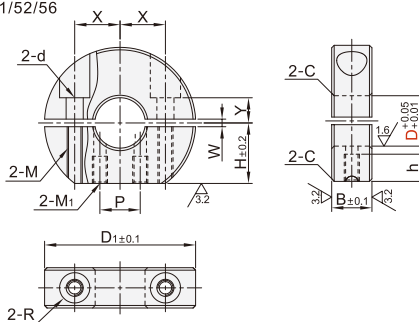
分离型 SBB51/52/56
