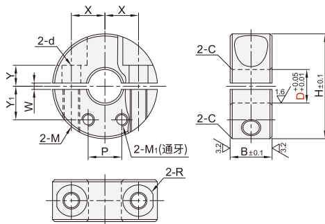
分离型 SBU51/52/56
