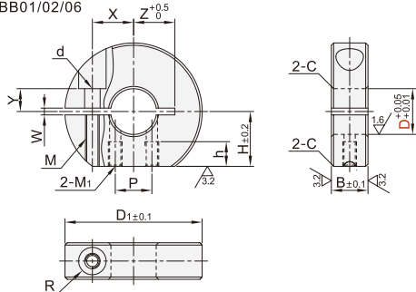
开口型 SBB01/02/06
