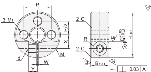
三螺孔锁紧型 SBL51/52/56
