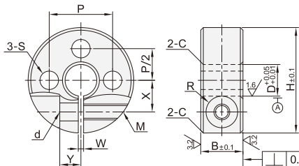
三孔锁紧型 SBL01/02/06
