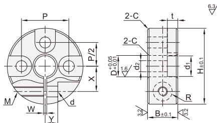
三沉孔锁紧型 SBF71/72/76
