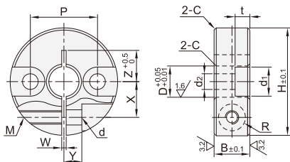
双沉孔锁紧型 SBF41/42/46
