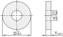
垫圈 SAA41
