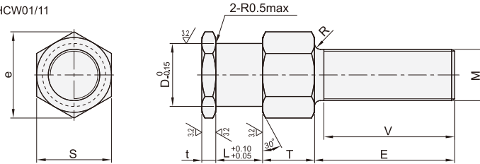
外螺纹型 HHCW01/11
