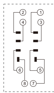
接线图
