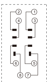
接线图
