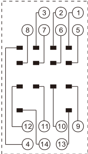
接线图
