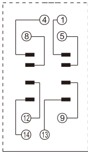
接线图
