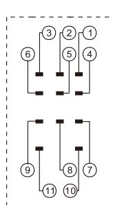
接线图
