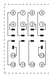
接线图
