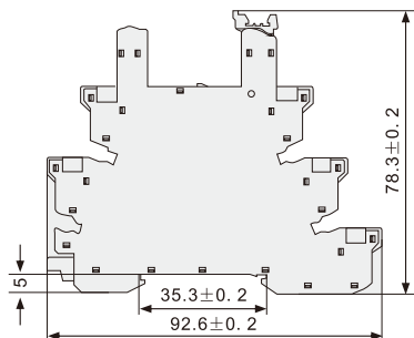
外形及安装尺寸 JDUA31
