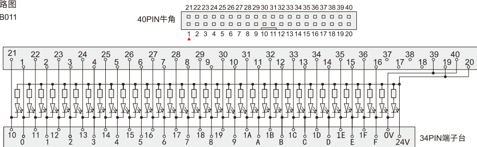
电路图
