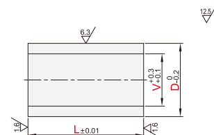
精密型 EYCJ31/32/33/34/35/36/37/38
