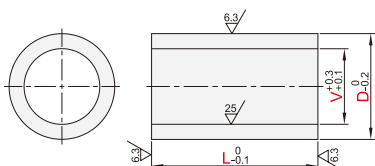
经济型 E-EYCJ01/02/03
