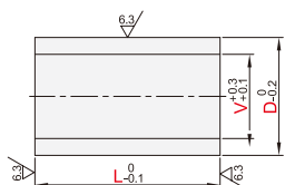
普通型 EYCJ01/02/07/11/12/13/ 14/15/16/17/18
