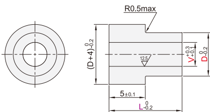
内径固定 EYCK01/02/07/08
